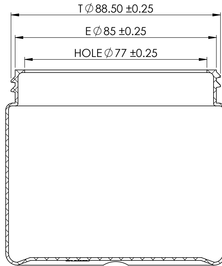
SECTION A-A
