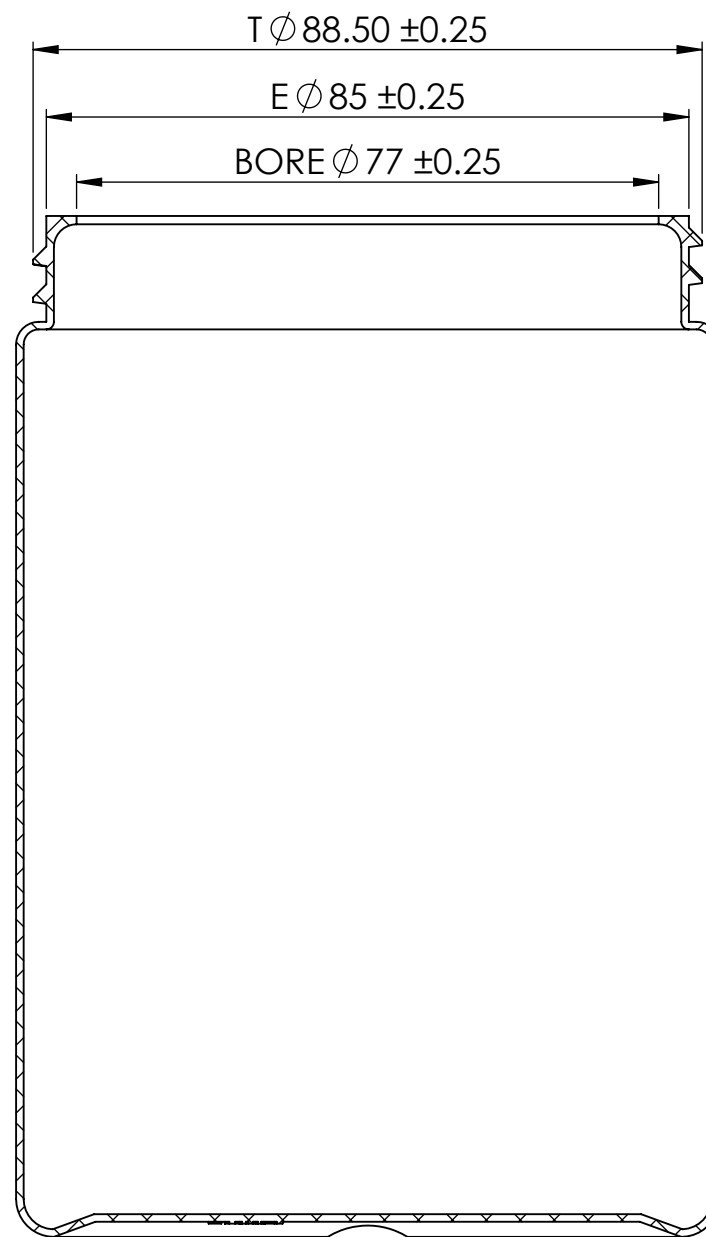
SECTION A-A
