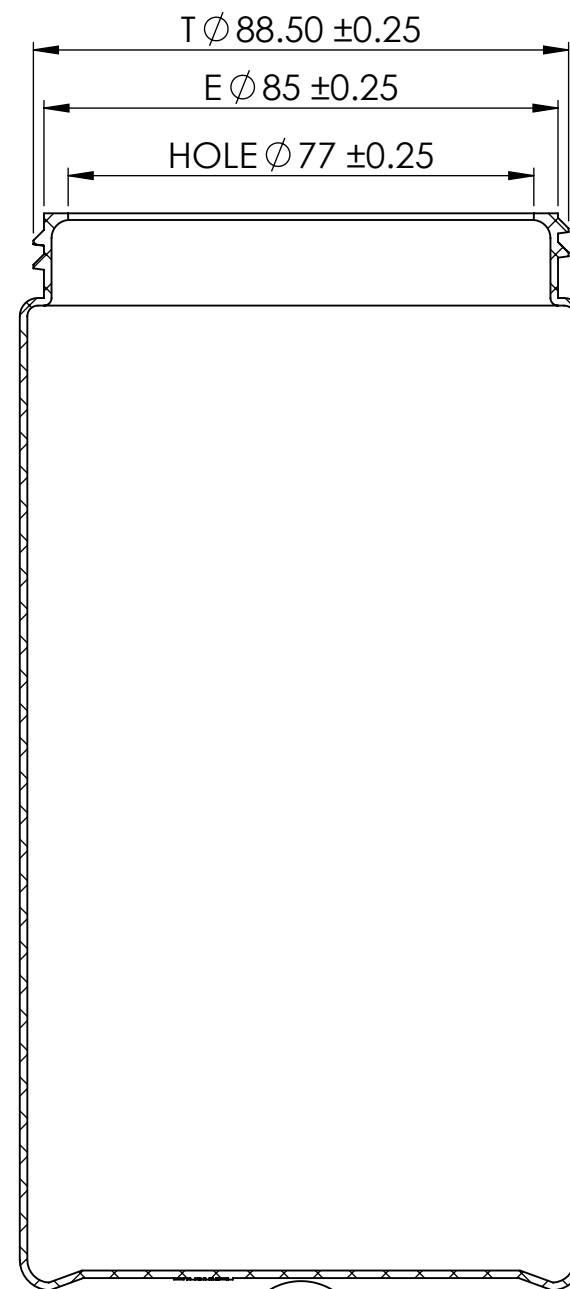
SECTION A-A
